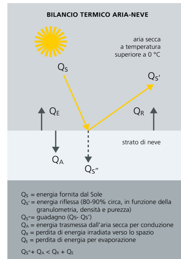
Fig. 7 Schema del bilancio termico aria-neve
