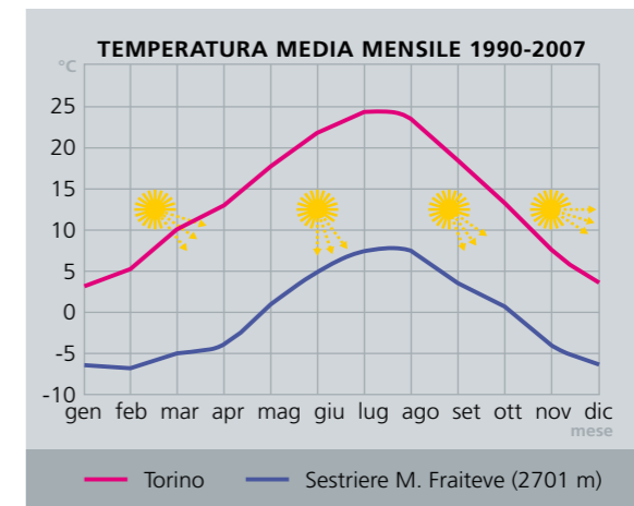
Fig. 6 Andamento annuale medio della temperatura in una stazione di pianura e una di vetta
